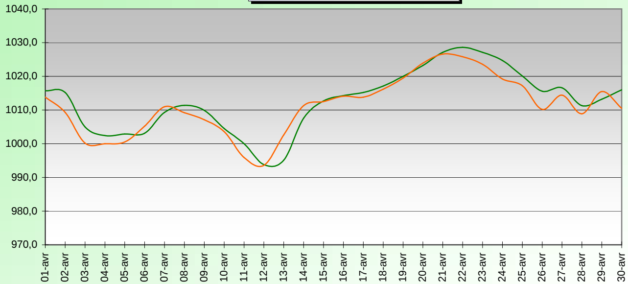
PRESSION RELATIVE (hPa) AVRIL 2002
