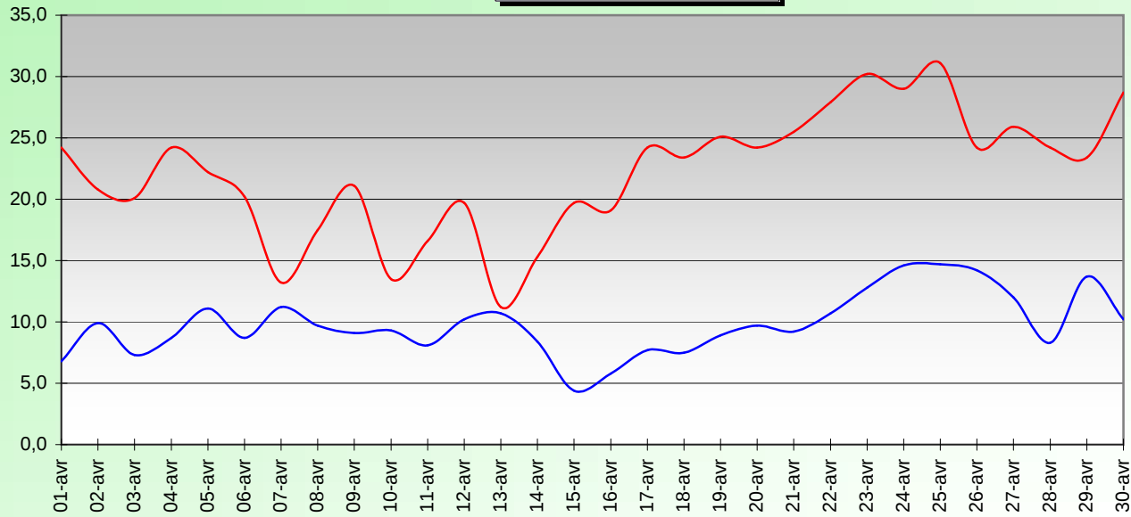
TEMPERATURE (°C) AVRIL 2002
