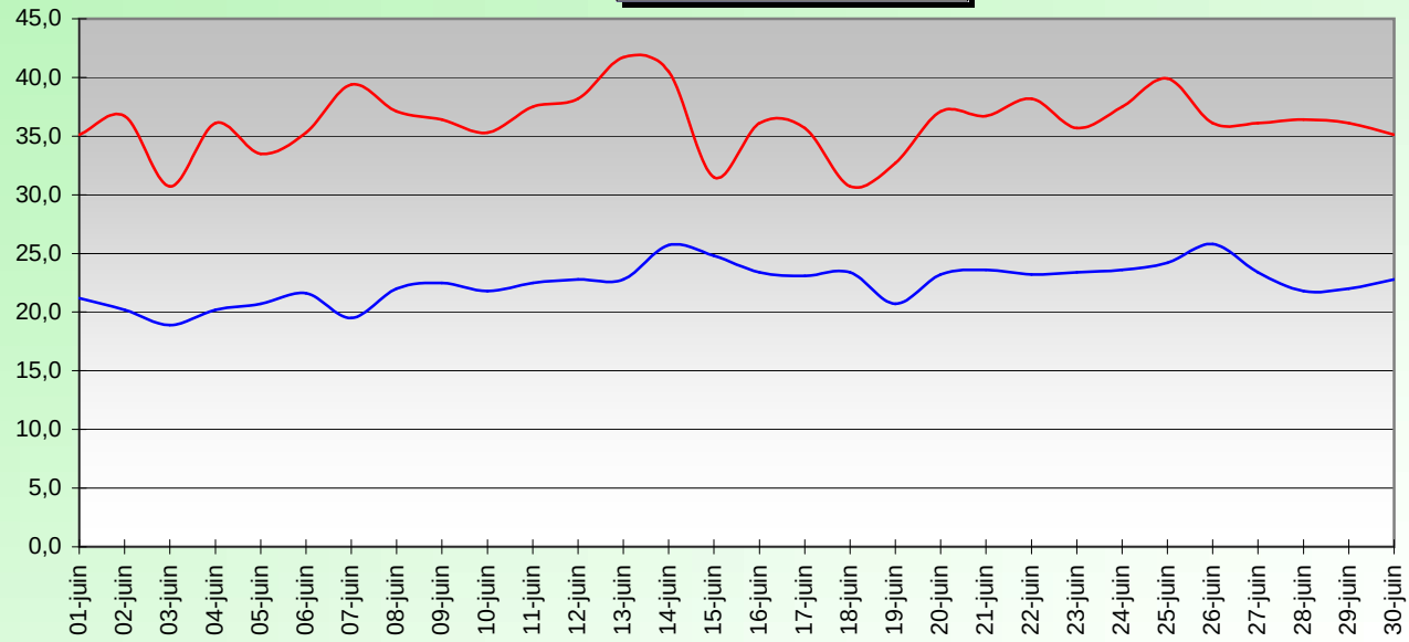
TEMPERATURE (°C) JUIN 2003
