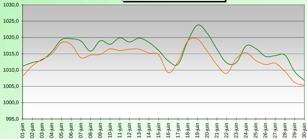
PRESSION RELATIVE (hPa) JUIN 2003
