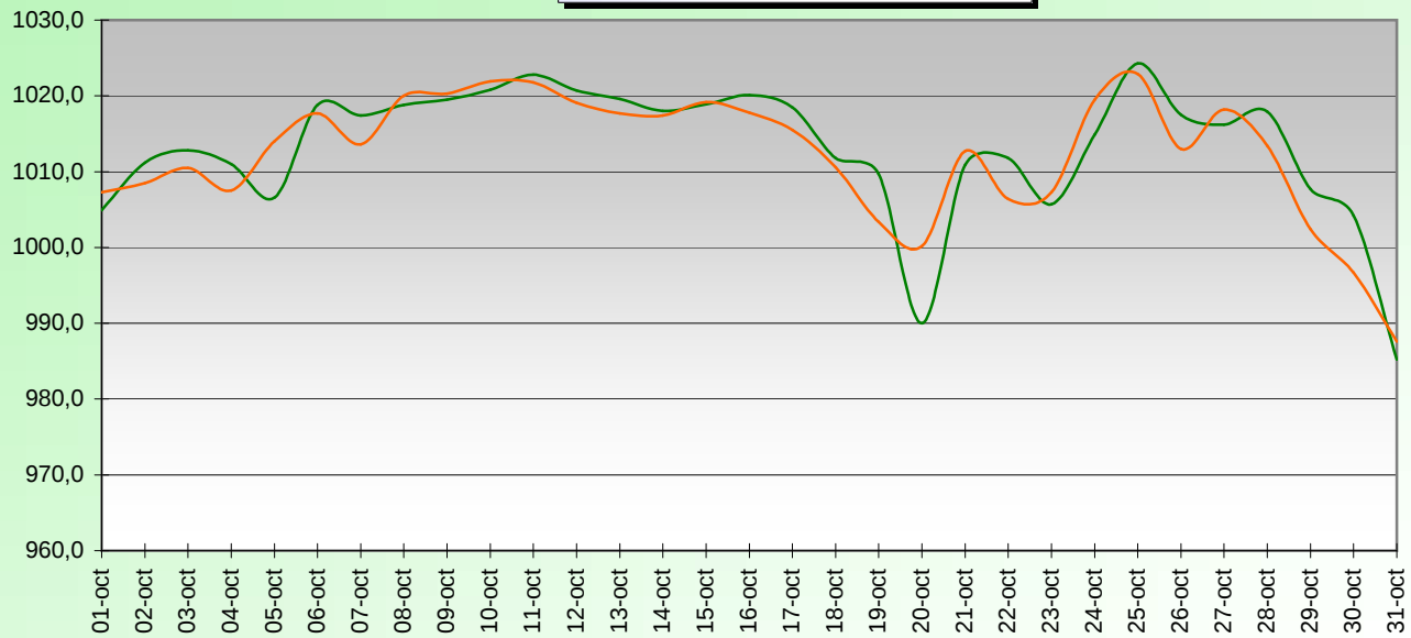
PRESSION RELATIVE (hPa) OCTOBRE 2003
