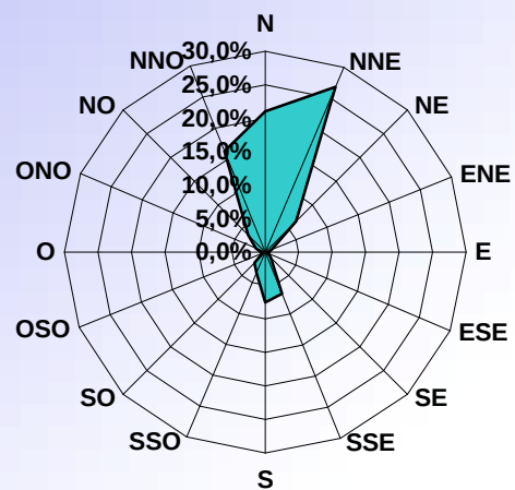
DISTRIBUTION ORIENTATION DU VENT MARS 2004
