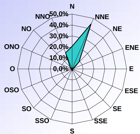
DISTRIBUTION ORIENTATION DU VENT NOVEMBRE 2004
