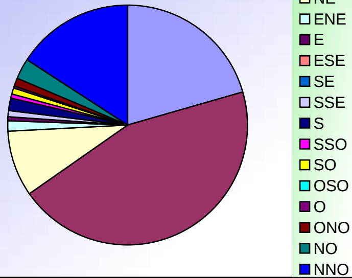
ORIENTATIONS DES VENTS NOVEMBRE 2004
