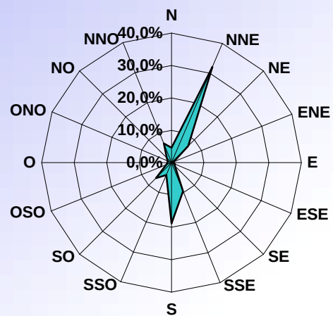
DISTRIBUTION ORIENTATION DU VENT AVRIL 2005
