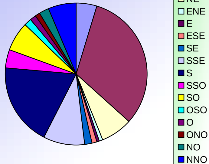
ORIENTATIONS DES VENTS AVRIL 2005
