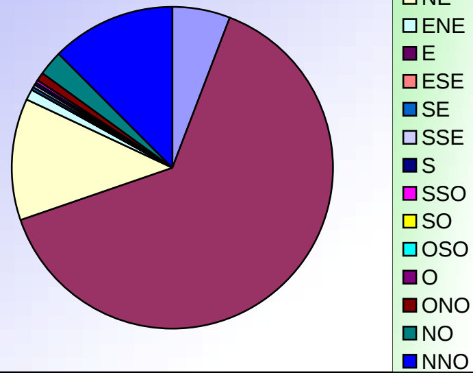
ORIENTATIONS DES VENTS FEVRIER 2005
