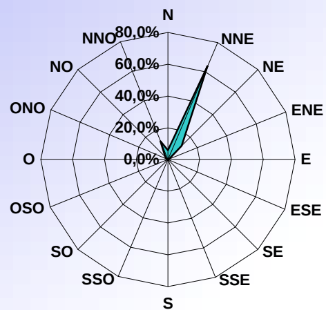
DISTRIBUTION ORIENTATION DU VENT FEVRIER 2005
