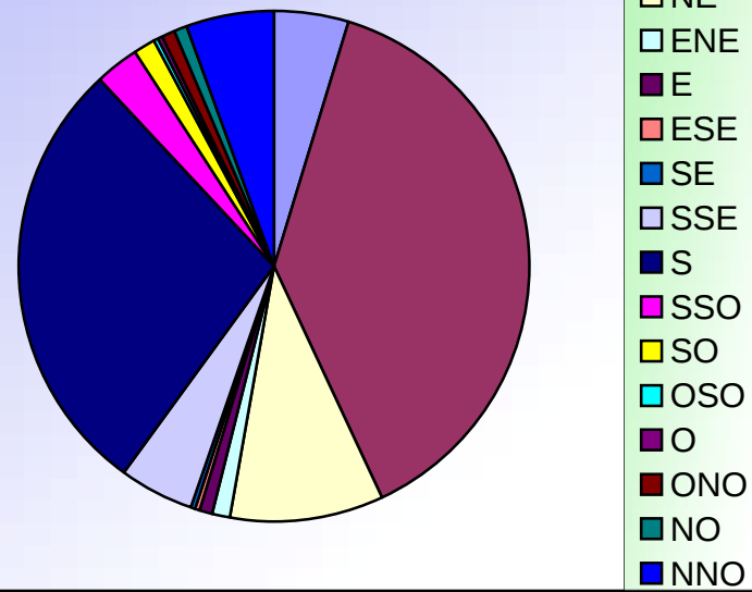
ORIENTATIONS DES VENTS JUILLET 2005
