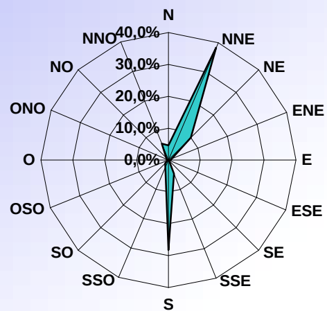
DISTRIBUTION ORIENTATION DU VENT JUILLET 2005
