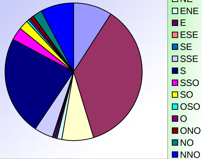
ORIENTATIONS DES VENTS JUN 2005
