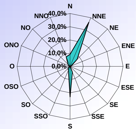
DISTRIBUTION ORIENTATION DU VENT JUN 2005
