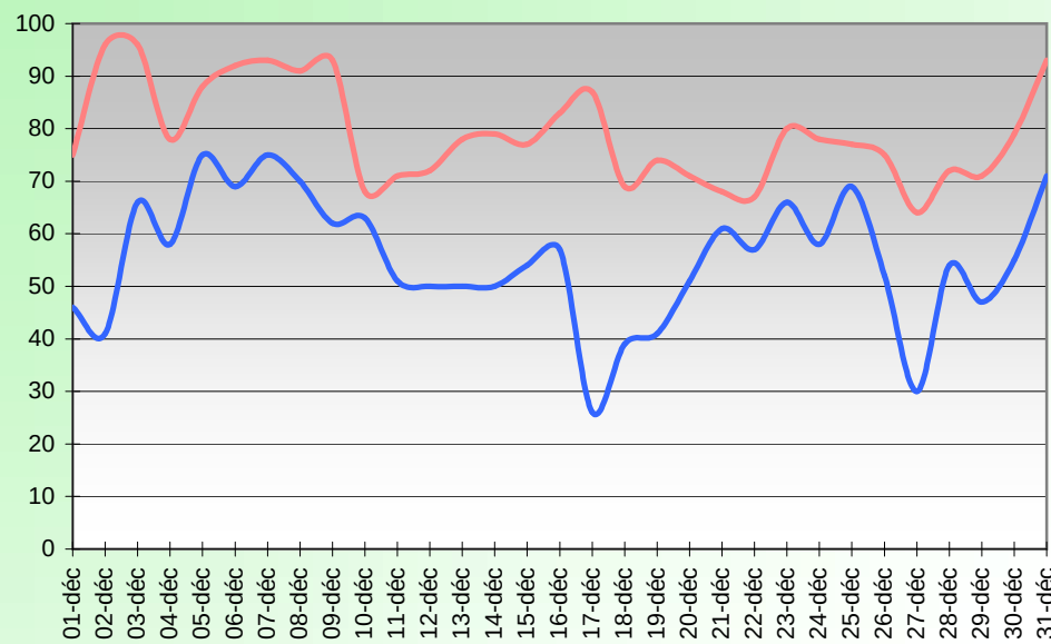
HUMIDITE RELATIVE (%) DECEMBRE 2005
