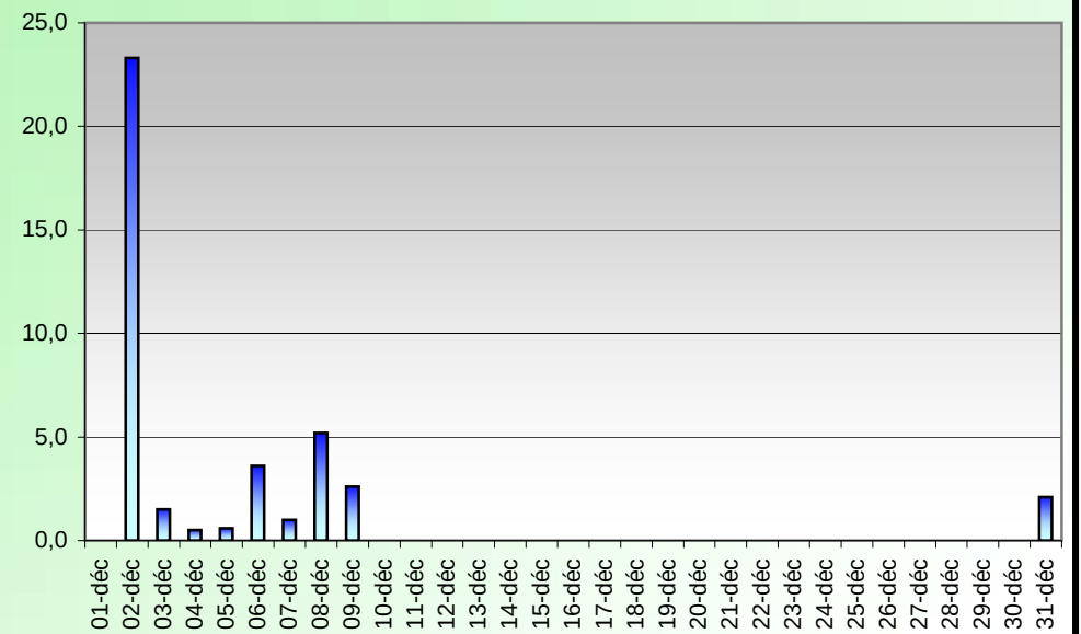
PRECIPITATIONS (mm) DECEMBRE 2005
