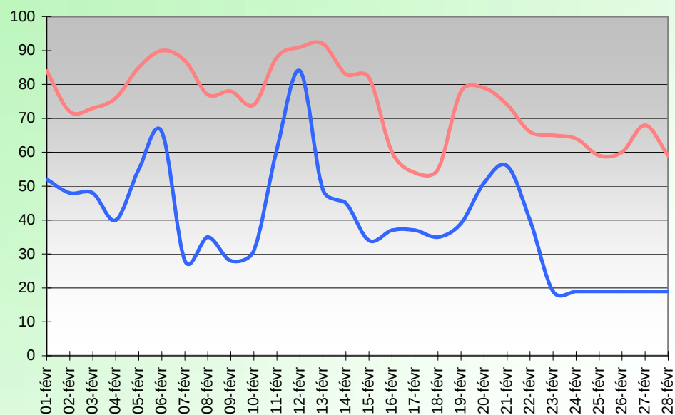
HUMIDITE RELATIVE (%) FEVRIER 2005
