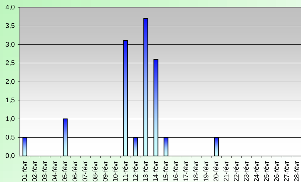
PRECIPITATIONS (mm) FEVRIER 2005
