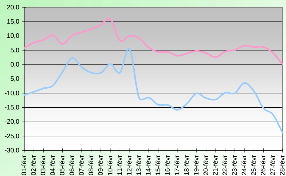
WINDCHILL (°C) FEVRIER 2005
