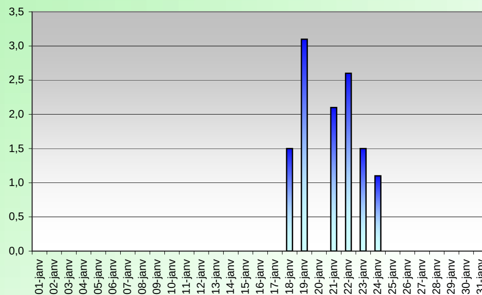
PRECIPITATIONS (mm) JANVIER 2005
