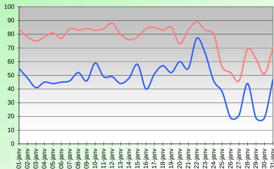
HUMIDITE RELATIVE (%) JANVIER 2005
