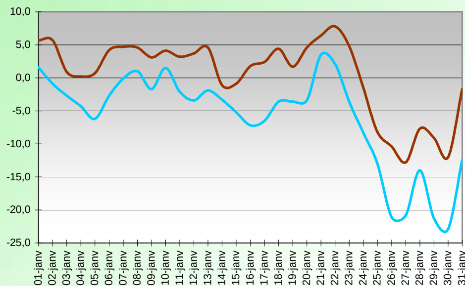
WINDCHILL (°C) JANVIER 2005
