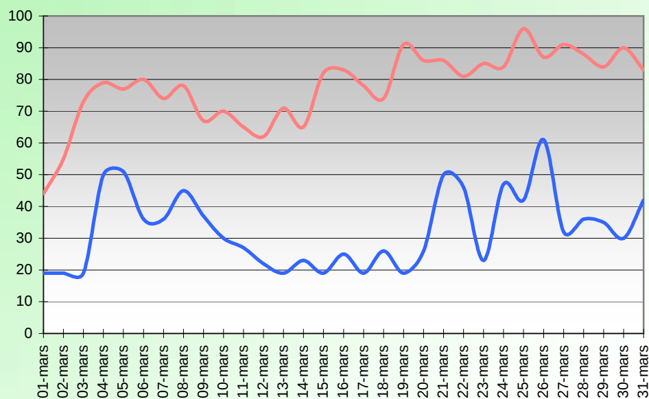
HUMIDITE RELATIVE (%) MARS 2005
