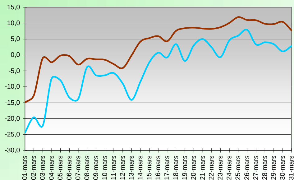
WINDCHILL (°C) MARS 2005
