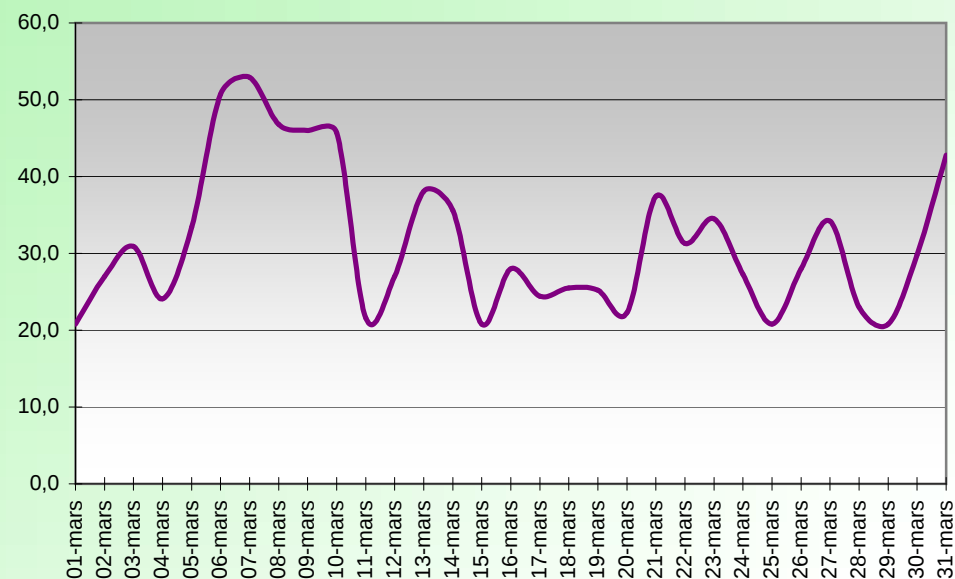
WINDCHILL (°C) MARS 2005
