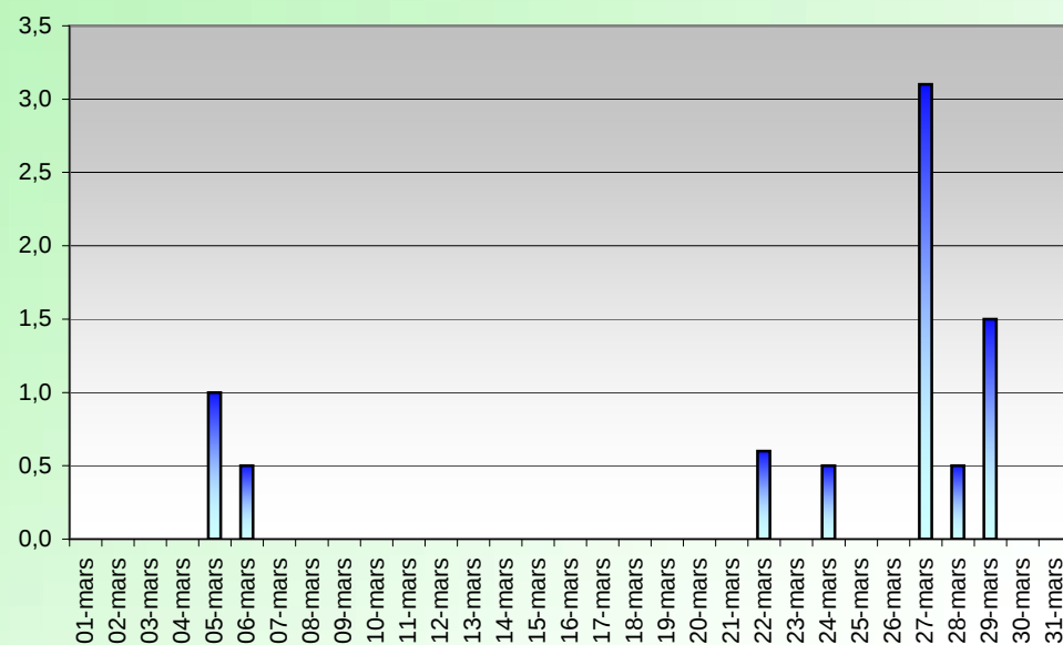
PRECIPITATIONS (mm) MARS 2005
