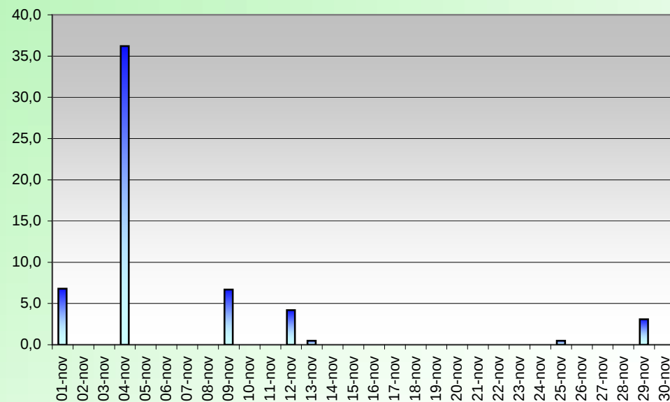
PRECIPITATIONS (mm) NOVEMBRE 2005
