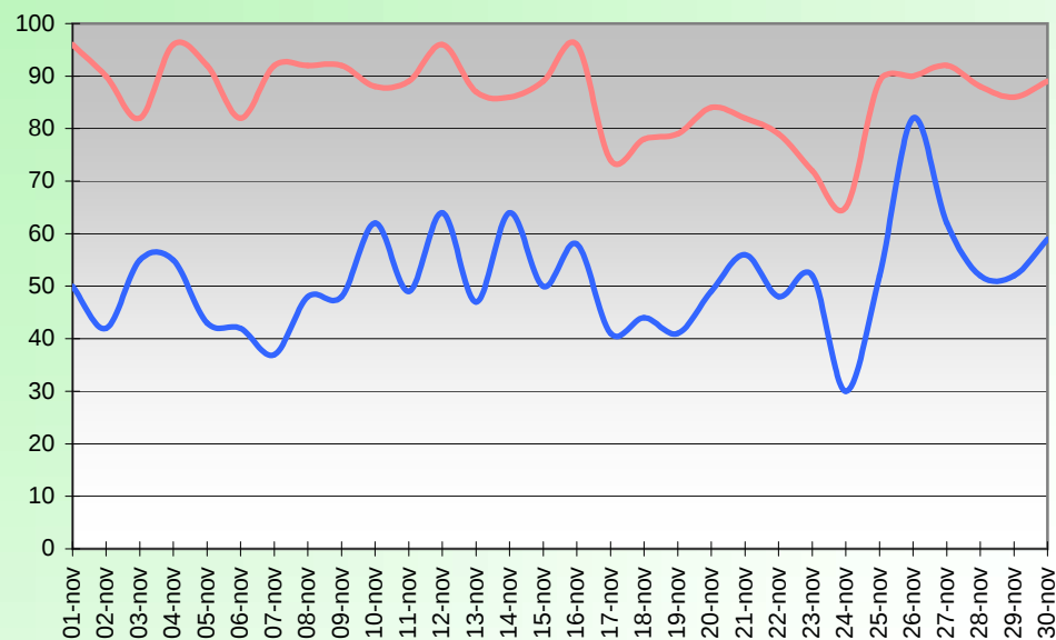
HUMIDITE RELATIVE (%) NOVEMBRE 2005
