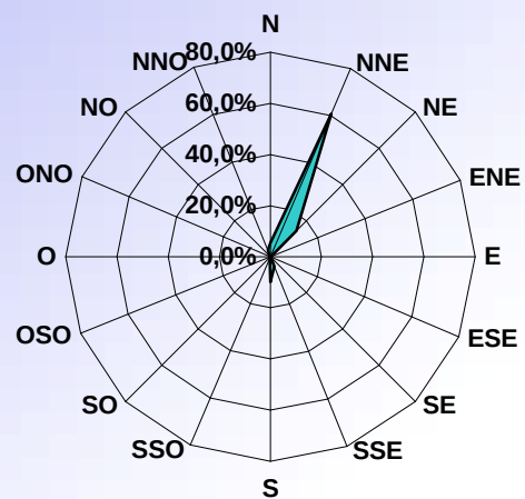
DISTRIBUTION ORIENTATION DU VENT AOUT 2006
