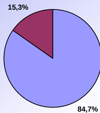
RAPPORT VENT NUL - VENT >0 AOUT 2006
