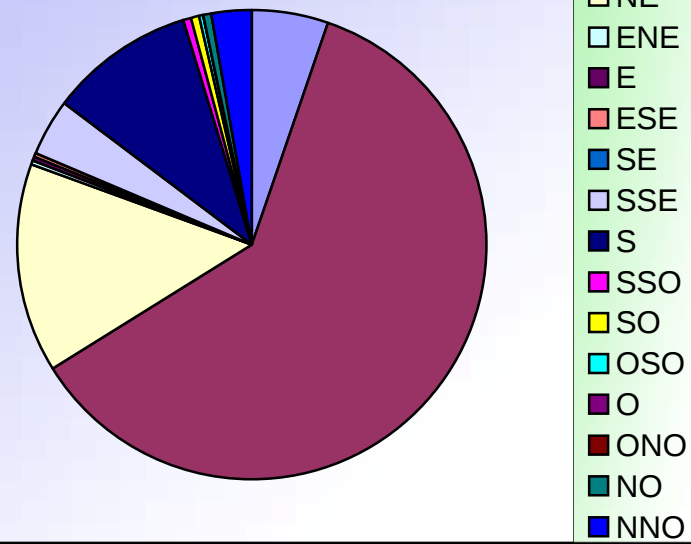
ORIENTATIONS DES VENTS AOUT 2006
