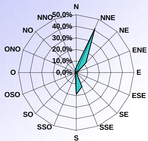
DISTRIBUTION ORIENTATION DU VENT JUILLET 2006
