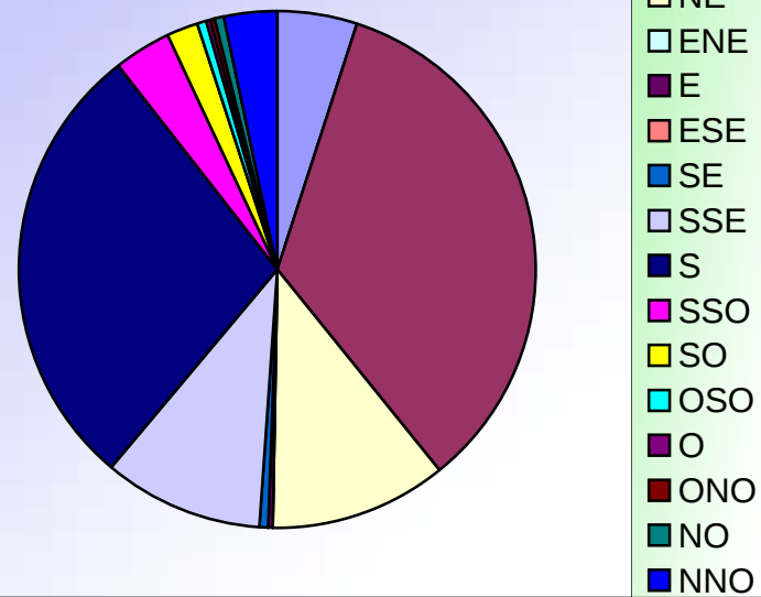
ORIENTATIONS DES VENTS JUN 2006
