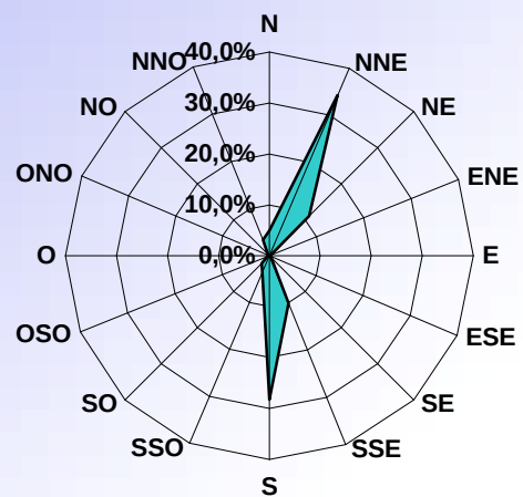
DISTRIBUTION ORIENTATION DU VENT JUN 2006
