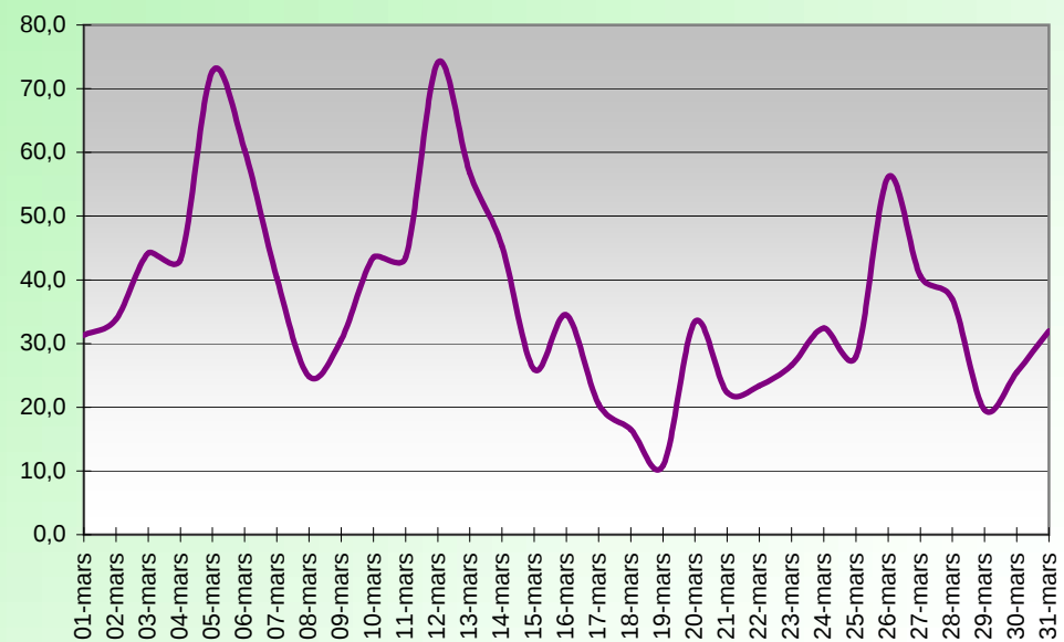
VENT (Km/H) MARS 2006
