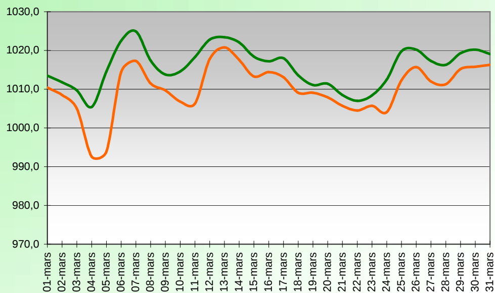
PRESSION RELATIVE (hPa) MARS 2006
