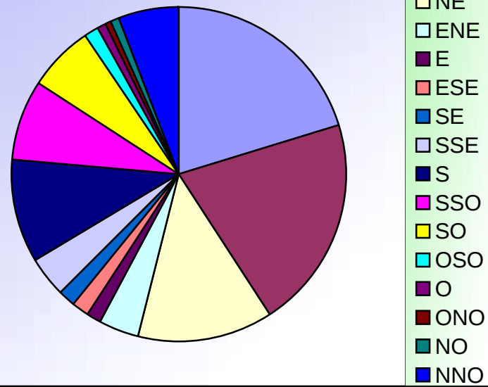
ORIENTATIONS DES VENTS AOUT 2007
