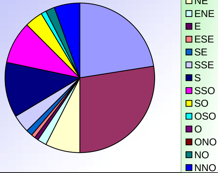
ORIENTATIONS DES VENTS JANVIER 2007
