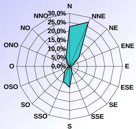
DISTRIBUTION ORIENTATION DU VENT JANVIER 2007
