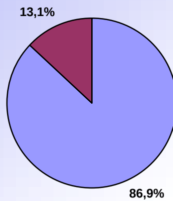
RAPPORT VENT NUL - VENT >0 JANVIER 2007
