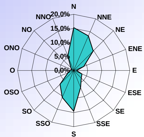
DISTRIBUTION ORIENTATION DU VENT JUN 2007
