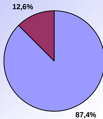
RAPPORT VENT NUL - VENT >0 JUN 2007
