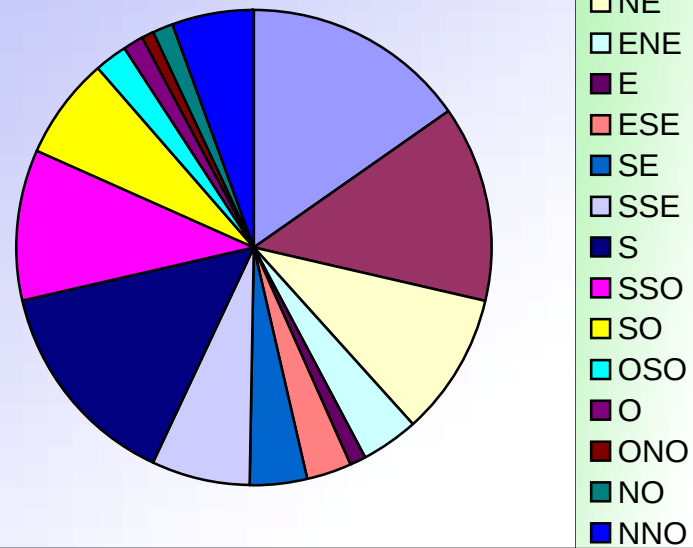
ORIENTATIONS DES VENTS JUN 2007
