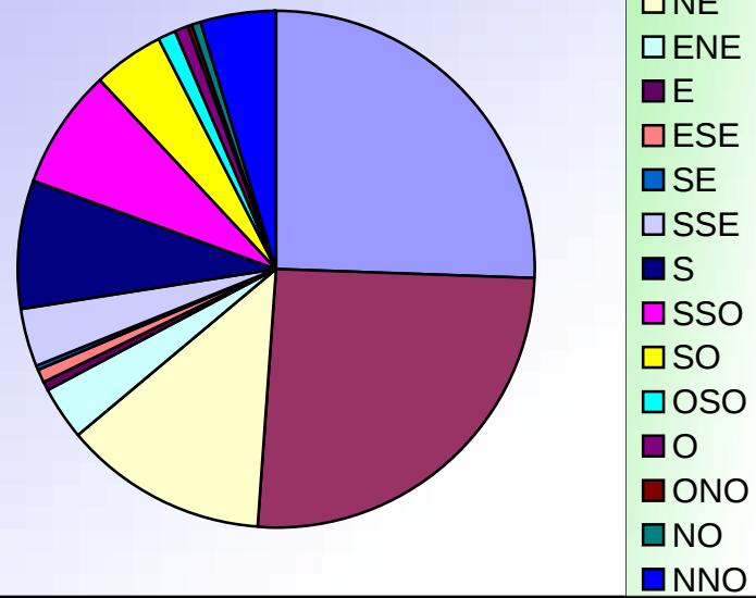
ORIENTATIONS DES VENTS SEPTEMBRE 2007
