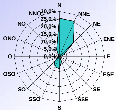
DISTRIBUTION ORIENTATION DU VENT SEPTEMBRE 2007
