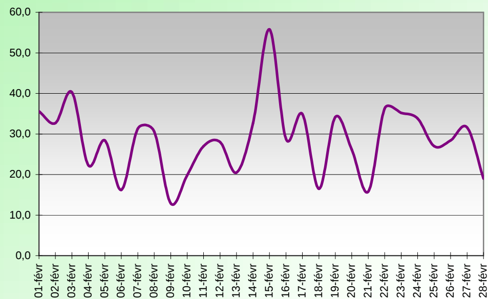
WINDCHILL (°C) FEVRIER 2007
