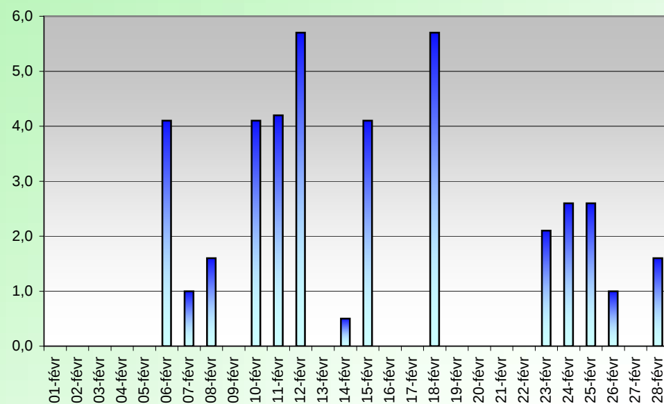
PRECIPITATIONS (mm) FEVRIER 2007
