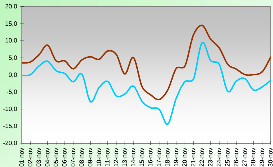
WINDCHILL (°C) NOVEMBRE 2007
