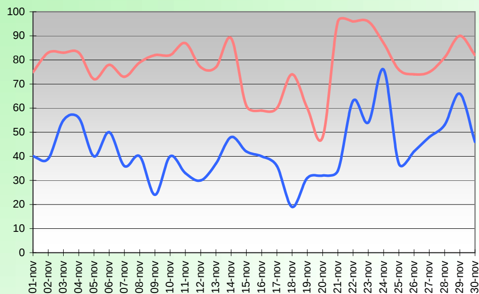
HUMIDITE RELATIVE (%) NOVEMBRE 2007
