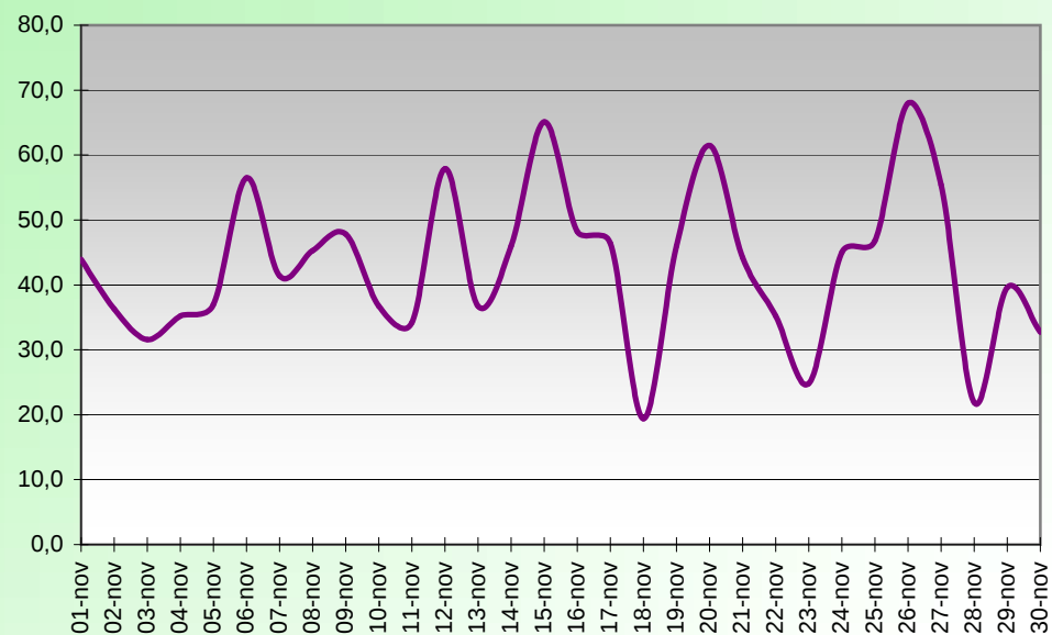
WINDCHILL (°C) NOVEMBRE 2007
