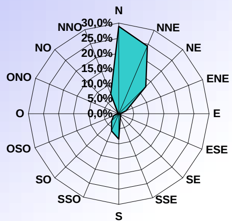
DISTRIBUTION ORIENTATION DU VENT AOUT 2008
