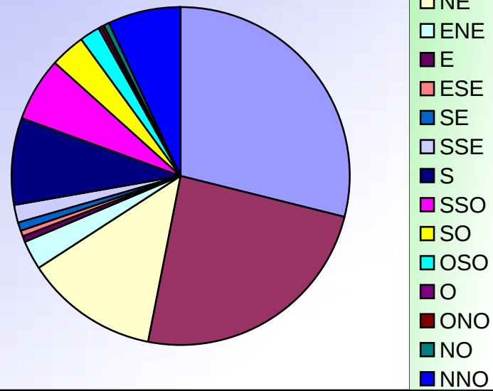
ORIENTATIONS DES VENTS AOUT 2008
