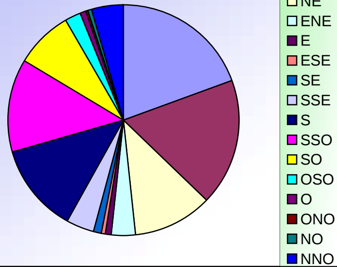
ORIENTATIONS DES VENTS AVRIL 2008
