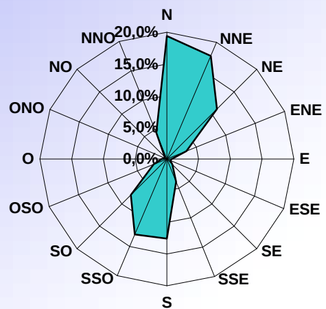
DISTRIBUTION ORIENTATION DU VENT AVRIL 2008
