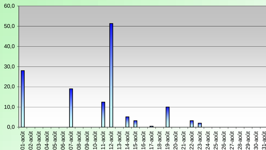
PRECIPITATIONS (mm) AOÛT 2008
