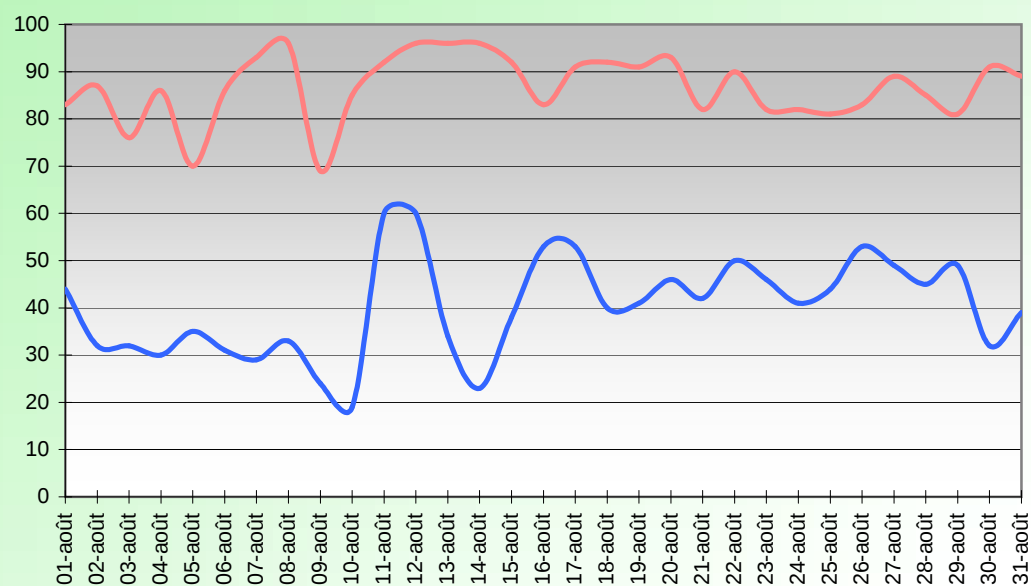
HUMIDITE RELATIVE (%) AOÛT 2008
