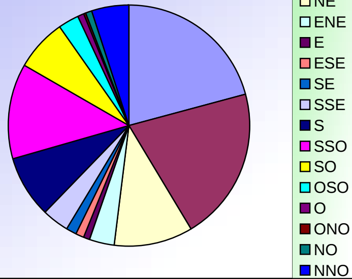
ORIENTATIONS DES VENTS DECEMBRE 2009
