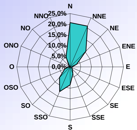
DISTRIBUTION ORIENTATION DU VENT DECEMBRE 2009
