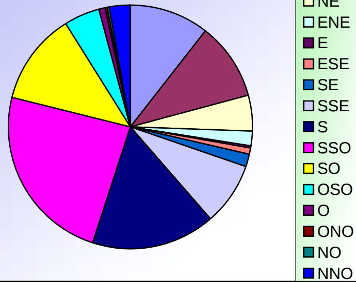
ORIENTATIONS DES VENTS NOVEMBRE 2009
