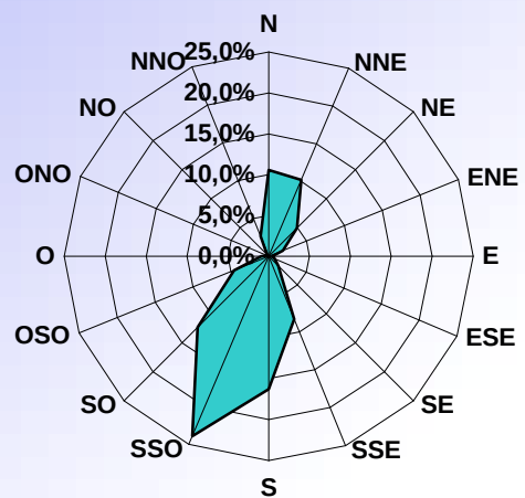
DISTRIBUTION ORIENTATION DU VENT NOVEMBRE 2009
