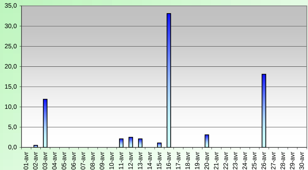
PRECIPITATIONS (mm) AVRIL 2009
