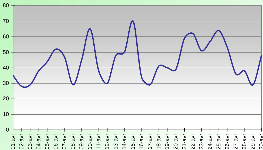
RAFALE MAXI (Km/H) AVRIL 2009
