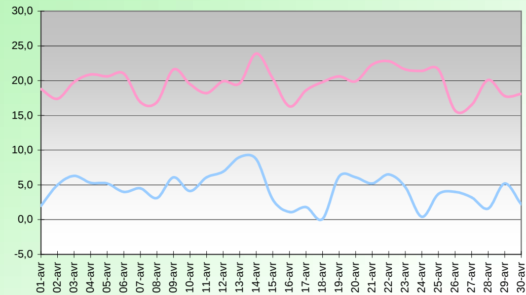
WINDCHILL (°C) AVRIL 2009
