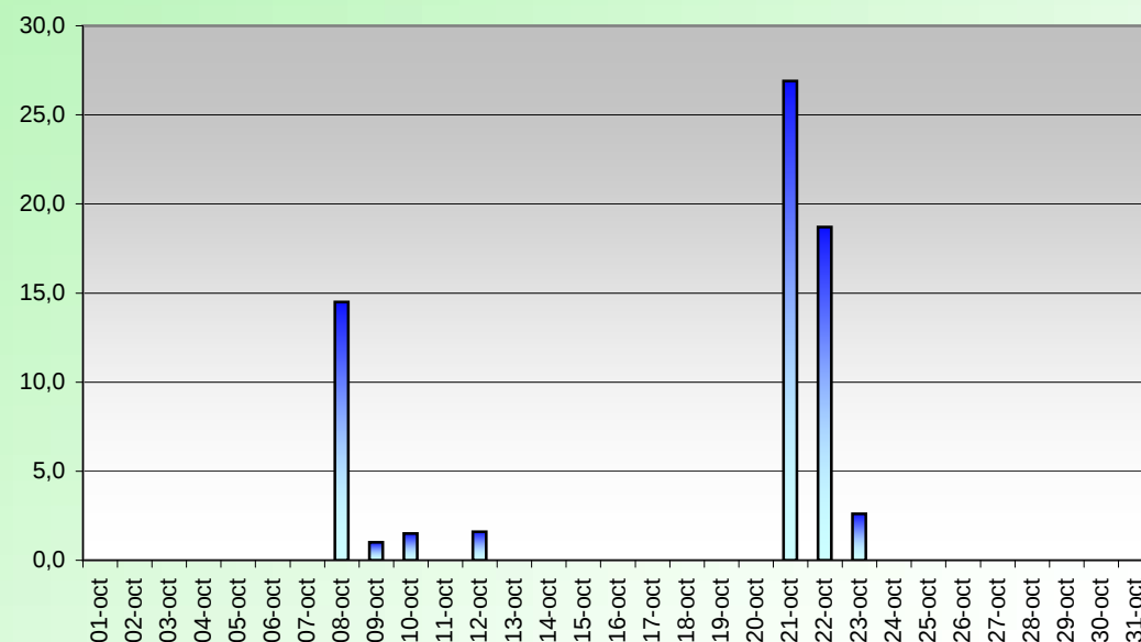
PRECIPITATIONS (mm) OCTOBRE 2009
