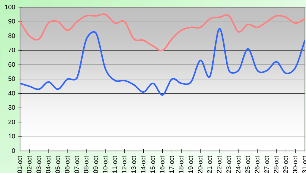
HUMIDITE RELATIVE (%) OCTOBRE 2009
