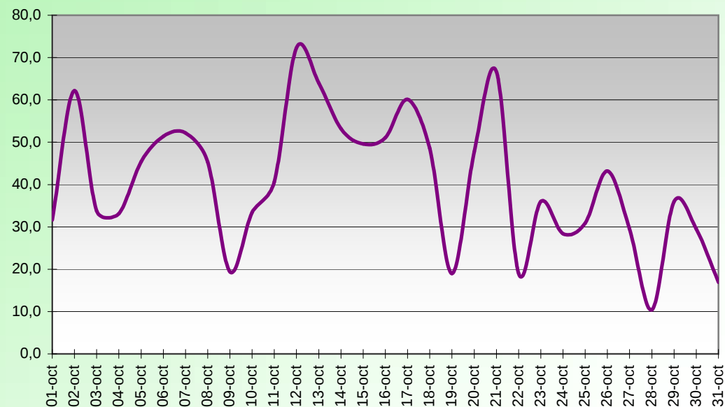
WINDCHILL (°C) OCTOBRE 2009
