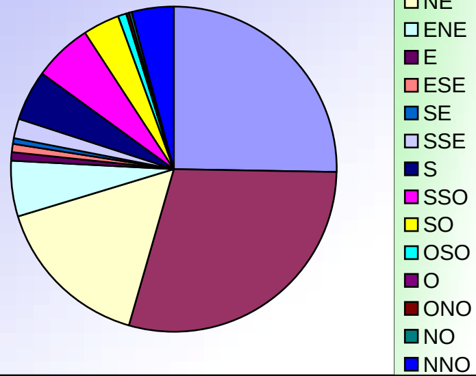
ORIENTATIONS DES VENTS JANVIER 2010
