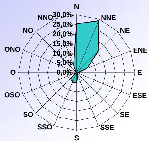
DISTRIBUTION ORIENTATION DU VENT JANVIER 2010
