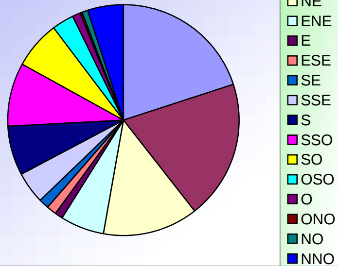
ORIENTATIONS DES VENTS JUILLET 2010
