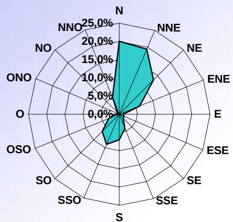
DISTRIBUTION ORIENTATION DU VENT JUILLET 2010
