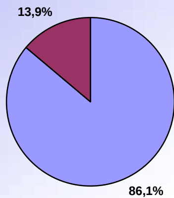
RAPPORT VENT NUL - VENT >0 MARS 2010
