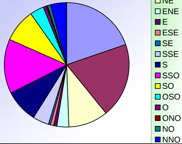
ORIENTATIONS DES VENTS MARS 2010
