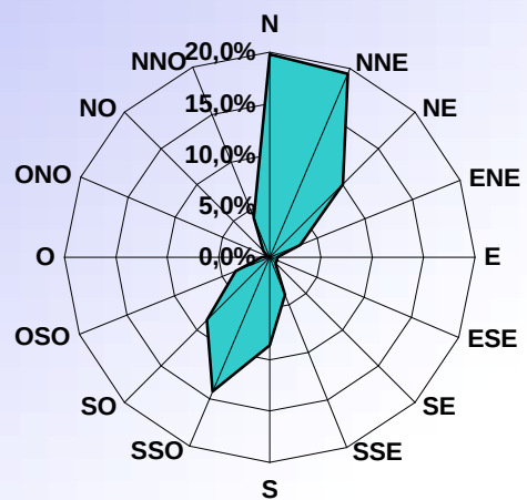
DISTRIBUTION ORIENTATION DU VENT MARS 2010
