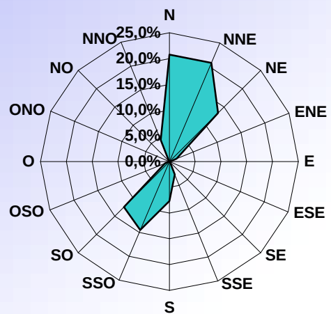
DISTRIBUTION ORIENTATION DU VENT NOVEMBRE 2010
