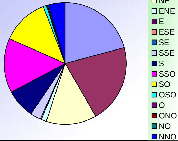
ORIENTATIONS DES VENTS NOVEMBRE 2010
