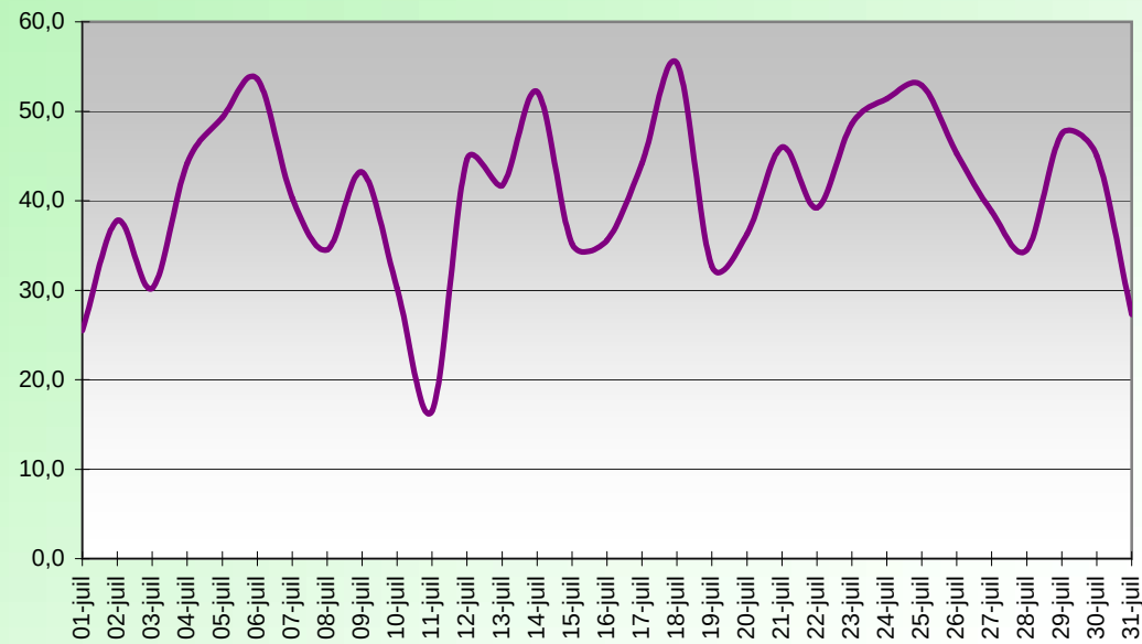
WINDCHILL (°C) JUILLET 2010
