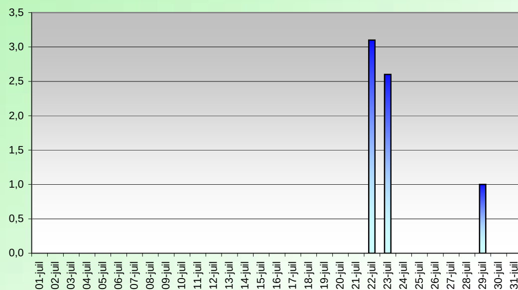
PRECIPITATIONS (mm) JUILLET 2010
