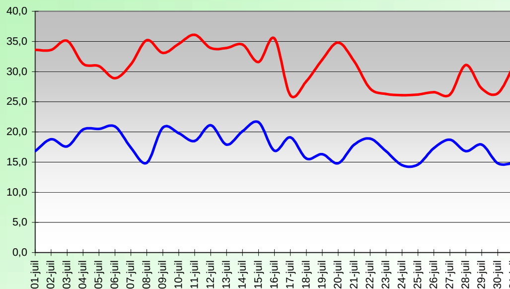
HUMIDITE RELATIVE (%) JUILLET 2010
