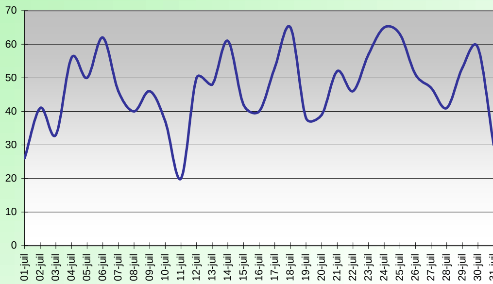
RAFALE MAXI (Km/H) JUILLET 2010
