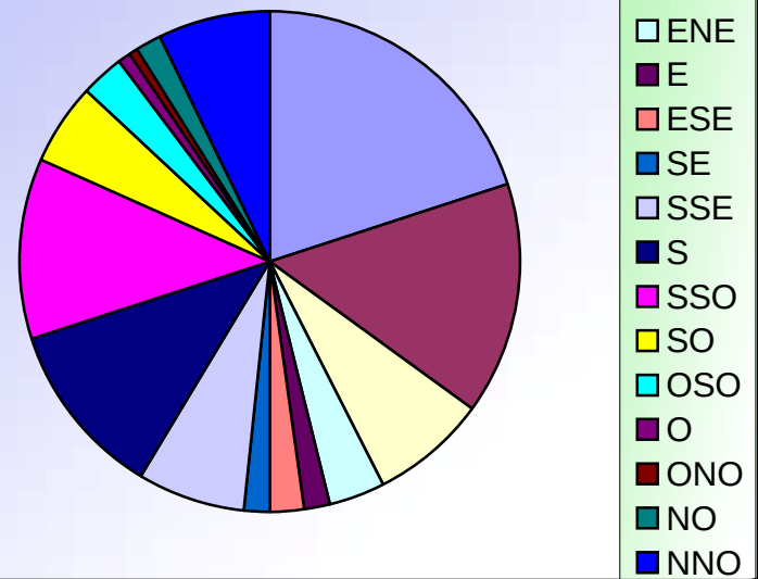
ORIENTATIONS DES VENTS DECEMBRE 2011
