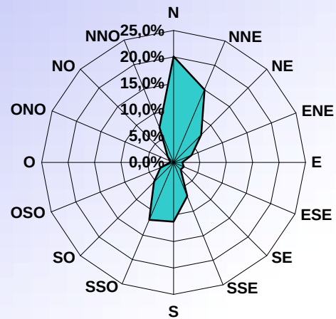
DISTRIBUTION ORIENTATION DU VENT DECEMBRE 2011
