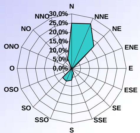
DISTRIBUTION ORIENTATION DU VENT FEVRIER 2011
