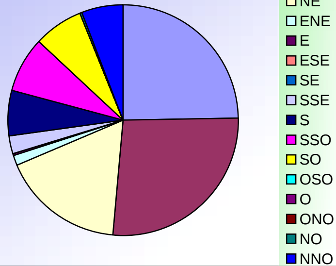
ORIENTATIONS DES VENTS FEVRIER 2011
