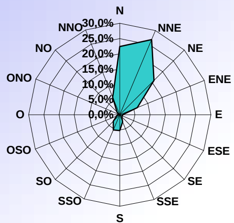
DISTRIBUTION ORIENTATION DU VENT JUILLET 2011
