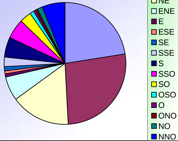
ORIENTATIONS DES VENTS JUILLET 2011
