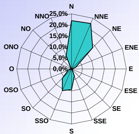
DISTRIBUTION ORIENTATION DU VENT SEPTEMBRE 2011
