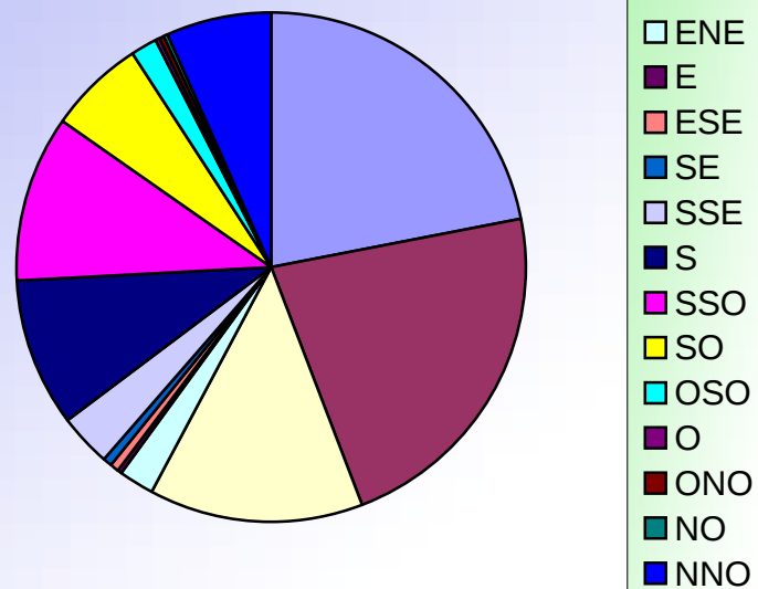
ORIENTATIONS DES VENTS SEPTEMBRE 2011
