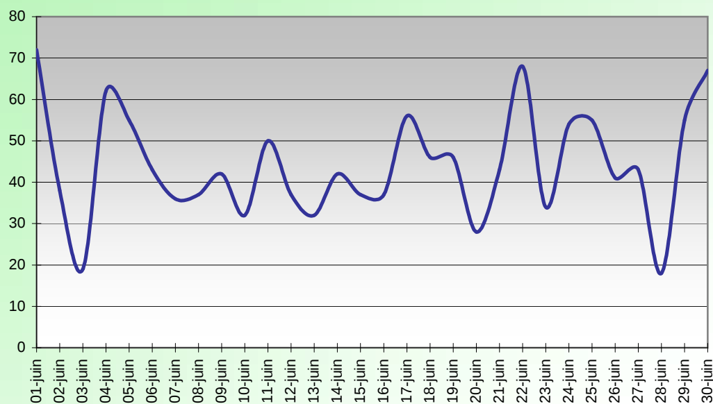
RAFALE MAXI (Km/H) JUIN 2011
