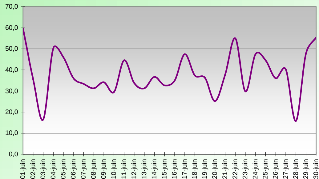
WINDCHILL (°C) JUIN 2011
