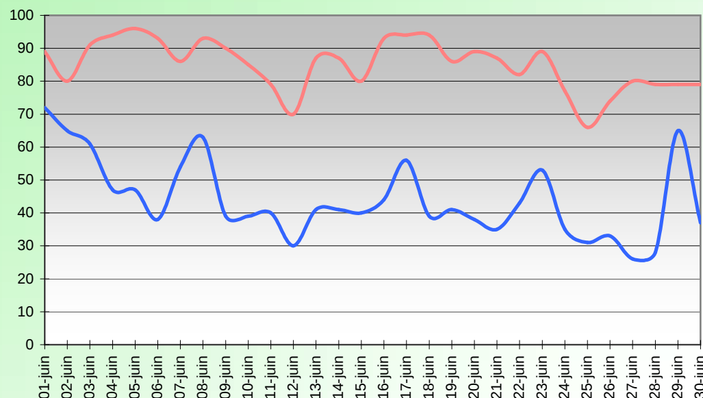
HUMIDITE RELATIVE (%) JUIN 2011
