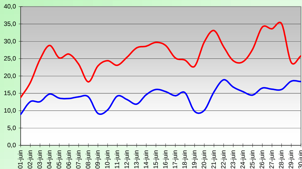
HUMIDITE RELATIVE (%) JUIN 2011
