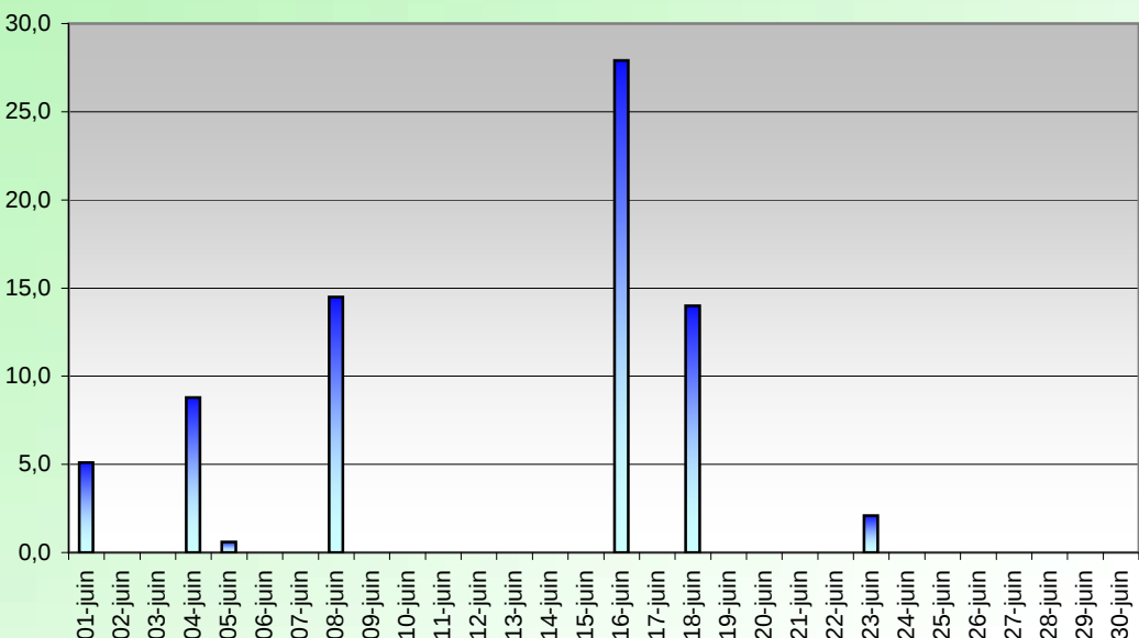
PRECIPITATIONS (mm) JUIN 2011
