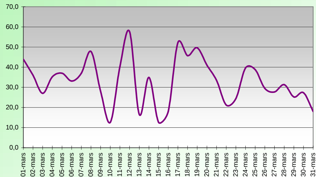
WINDCHILL (°C) MARS 2011
