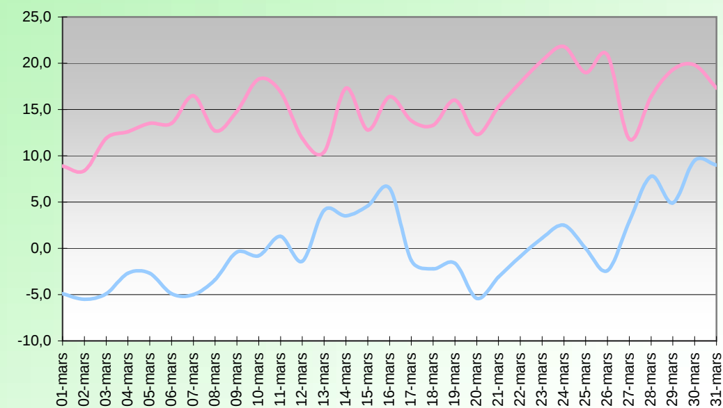
WINDCHILL (°C) MARS 2011
