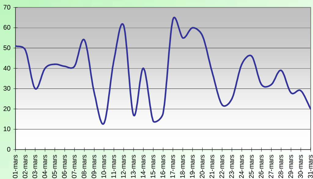
RAFALE MAXI (Km/H) MARS 2011
