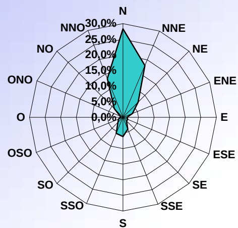
DISTRIBUTION ORIENTATION DU VENT JUILLET 2012
