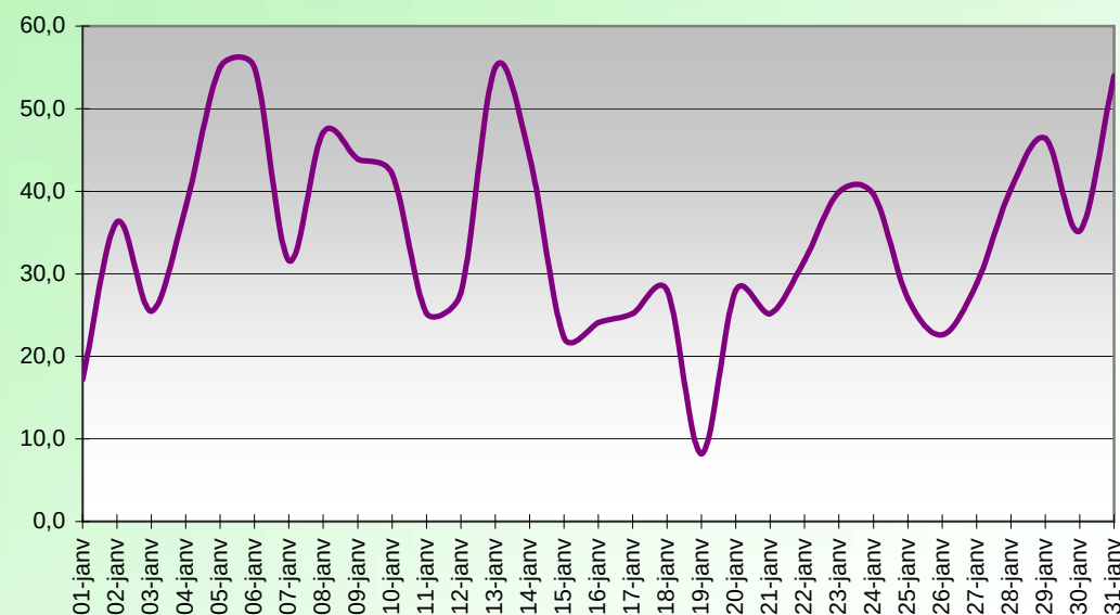
WINDCHILL (°C) JANVIER 2012
