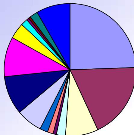
ORIENTATIONS DES VENTS ANNEE 2013
