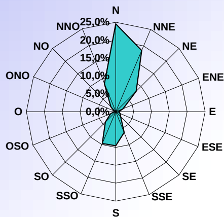
DISTRIBUTION ORIENTATION DU VENT ANNEE 2013
