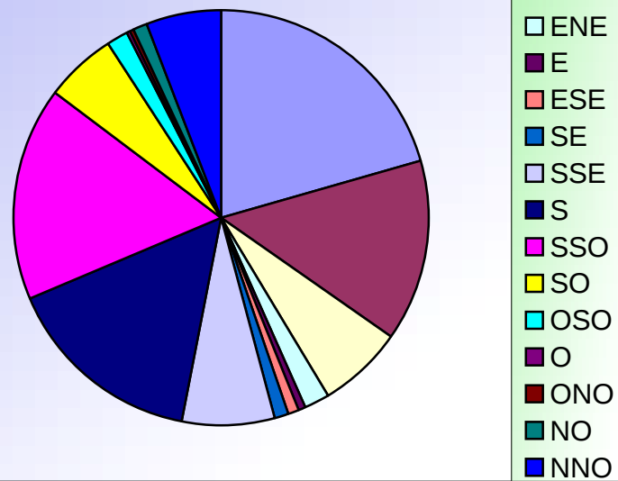
ORIENTATIONS DES VENTS DECEMBRE 2013
