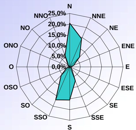
DISTRIBUTION ORIENTATION DU VENT DECEMBRE 2013
