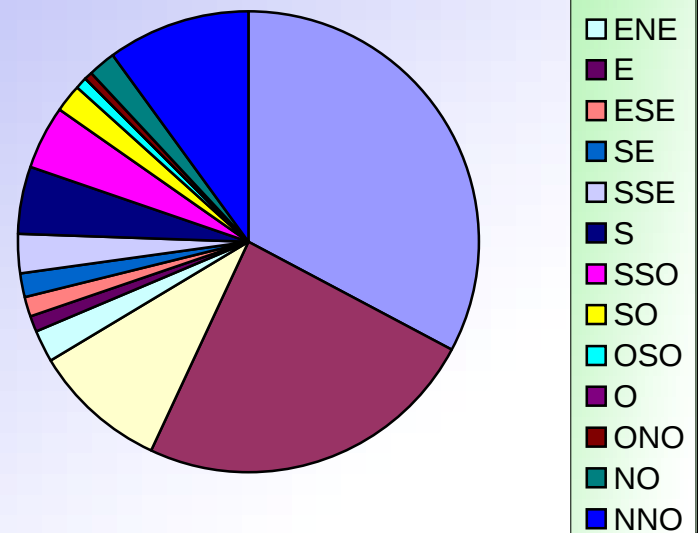
ORIENTATIONS DES VENTS JANVIER 2013
