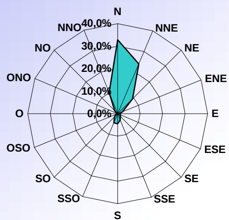
DISTRIBUTION ORIENTATION DU VENT JANVIER 2013
