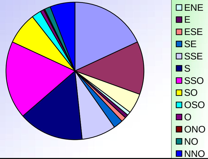
ORIENTATIONS DES VENTS OCTOBRE 2013
