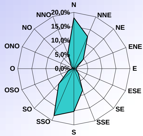
DISTRIBUTION ORIENTATION DU VENT OCTOBRE 2013
