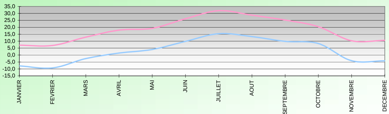
WINDCHILL (°C) 2013
