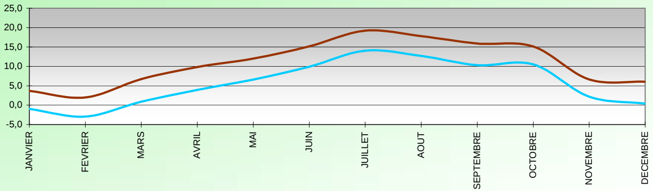
VENT (Km/H) 2013
