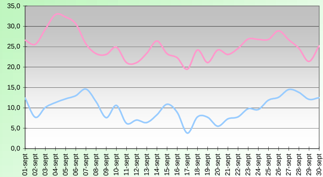
WINDCHILL (°C) SEPTEMBRE 2013
