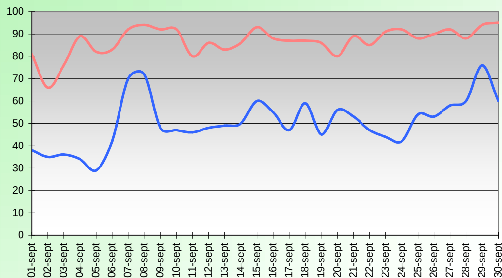
HUMIDITE RELATIVE (%) SEPTEMBRE 2013
