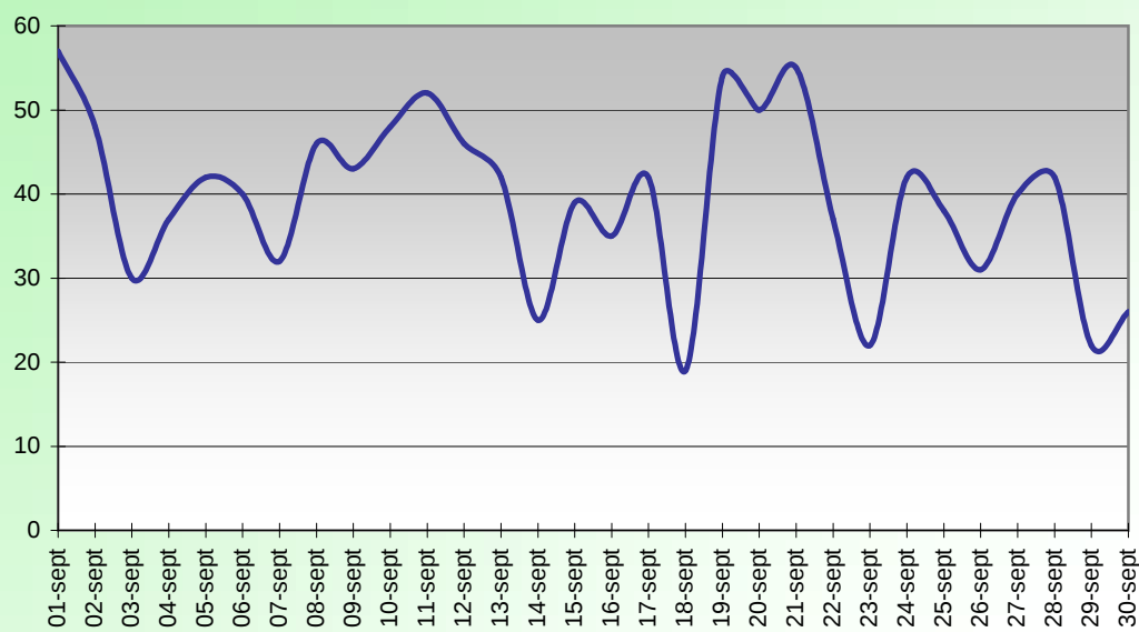
RAFALE MAXI (Km/H) SEPTEMBRE 2013
